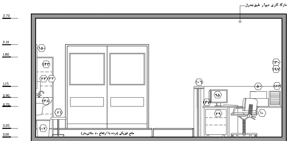
نقشه ۲-۱۴-۲- نمای ۲- مقیاس ۱:۵۰
