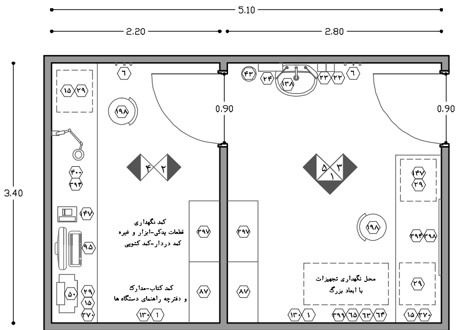
نقشه ۲-۱۰۷-۱- پلان نمونه‌ی اتاق کالیبراسیون و تعمیر در بخش‌های اعمال جراحی متوسط (۵ تا ۹ اتاق عمل) - مقیاس ۱:۵۰
