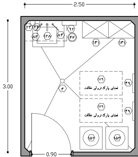
نقشه ۲-۲۵- پلان نمونه‌ی اتاق نظافت (روش نوین) مقیاس ۱:۵۰
