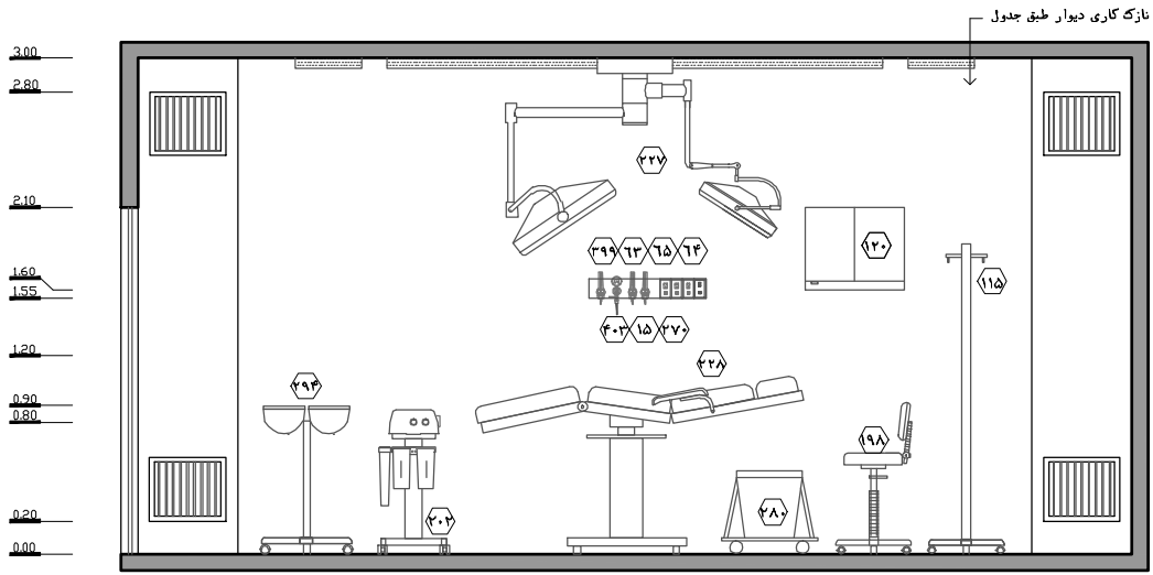
نقشه ۲-۱۴۸- نمای ۳- مقیاس ۱:۵۰
