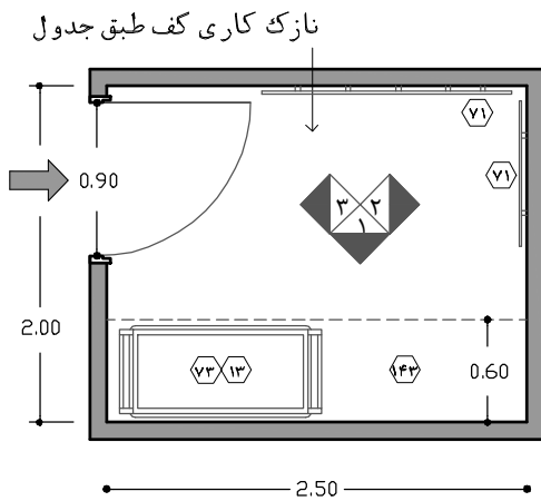
نقشه ۲-۶۹- پلان نمونه‌ی فضای نگهداری ملحفه و رخت تمیز در بخش‌های جراحی متوسط (۵ تا ۹ اتاق عمل) مقیاس ۱:۵۰
