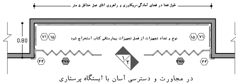
نقشه ۲-۵۹- پلان نمونه‌ی فضای پارک تجهیزات پزشکی آمادگی در بخش‌های جراحی کوچک (تا ۴ اتاق عمل) - مقیاس ۱:۵۰
