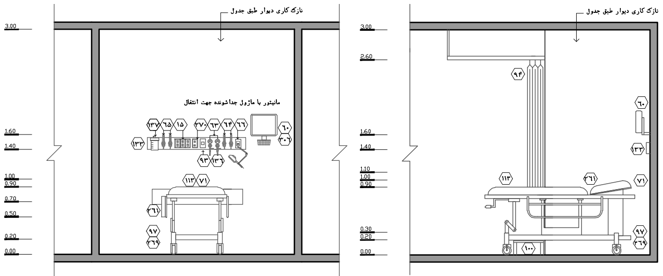
نقشه ۱-۴۶- نمای ۱- مقیاس ۱:۵۰
