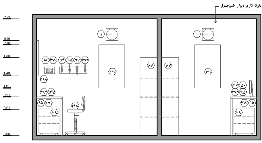
نقشه ۱۰۸-۲- نمای ۱- مقیاس ۱:۵۰
