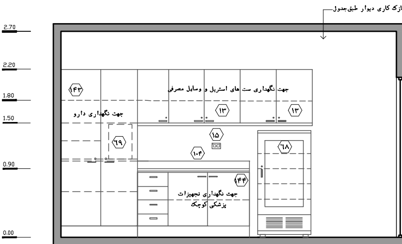
نقشه ۲-۵۷- نمای ۱- مقیاس ۱:۵۰
