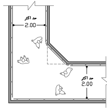
نقشه ۲-۱۸۰- ایجاد تمهیداتی همچون ایجاد شکستگی در کنج - مقیاس ۱:۱۰۰
