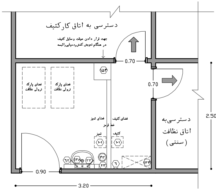
نقشه ۲-۳۴- پلان نمونه‌ی پیش‌ورودی اتاق‌های کثیف با دو فضای پارک در بخش‌های اعمال جراحی - مقیاس ۱:۵۰
