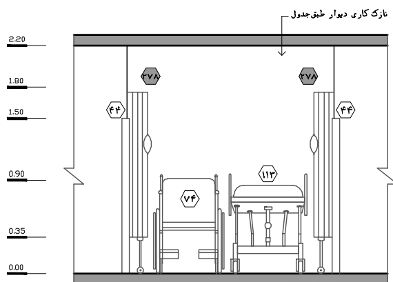
نقشه ۲-۲۰- نمای ۲- مقیاس ۱:۵۰
