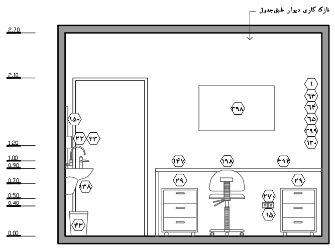
نقشه ۱۱۰-۲- نمای ۳- مقیاس ۱:۵۰
