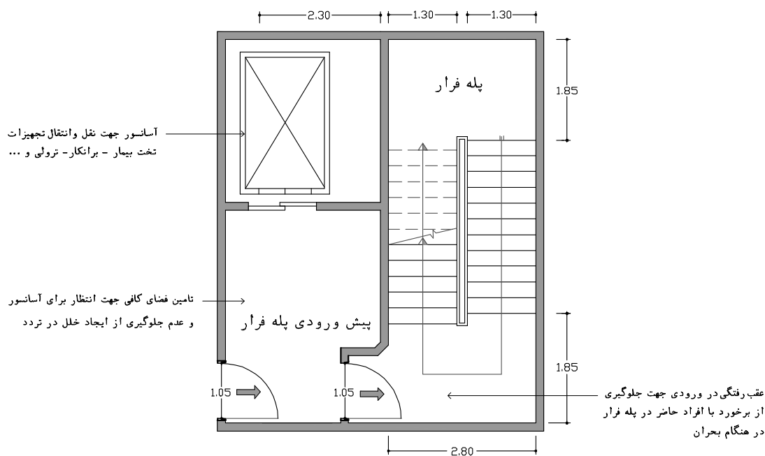
شکل ۲-۲۷- تعبیه‌ی آسانسور برانکاربر، در پیش‌ورودی پله‌های فرار
