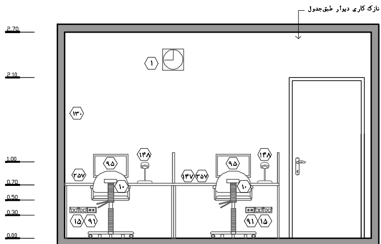
نقشه ۲-۱۲۸ - نمای ۲ - مقیاس ۱:۵۰
