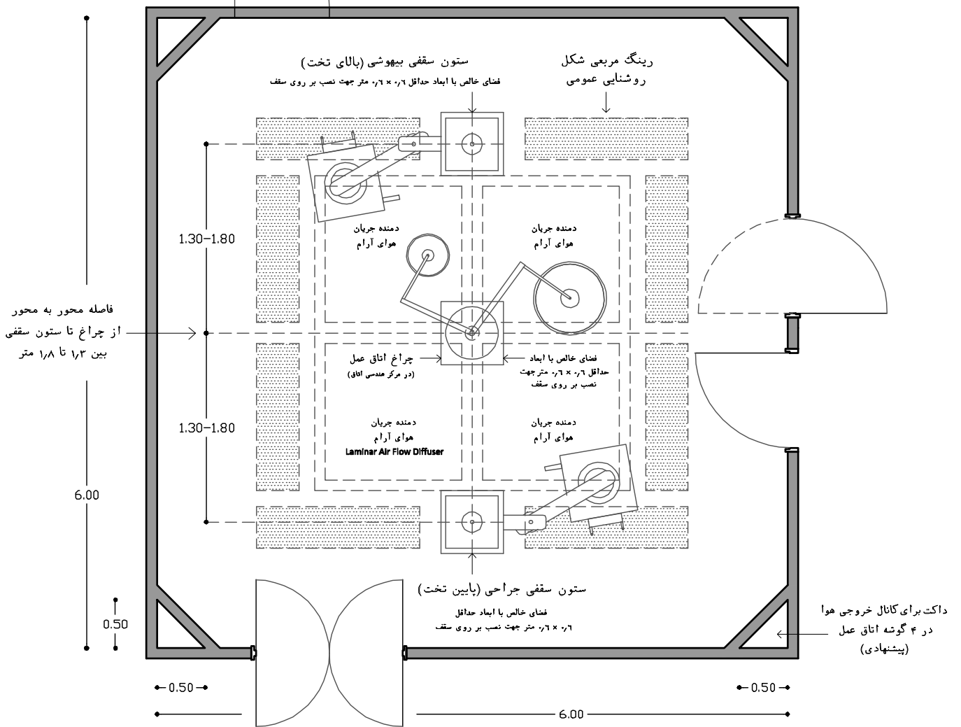
نقشه ۲-۱۵۰- پلان معکوس اتاق عمل جراحی کوچک - مقیاس ۱:۵۰
