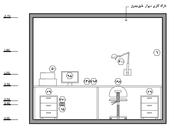
نقشه ۱۱۱-۲- نمای ۴- مقیاس ۱:۵۰
