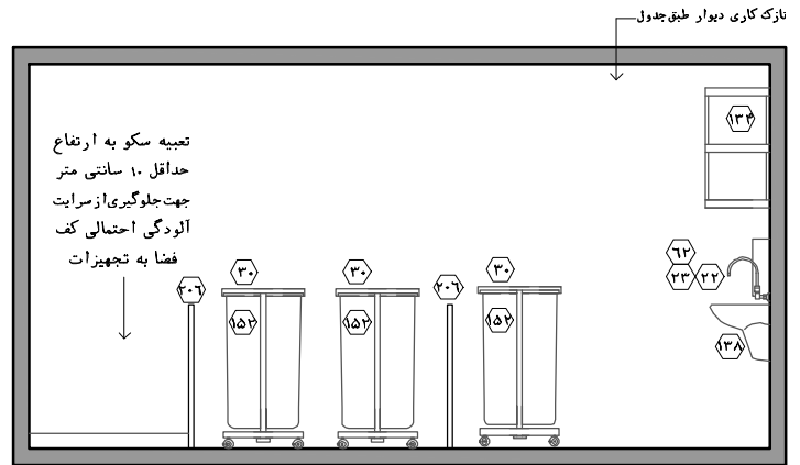
نقشه ۲-۴۱- نمای ۲- مقیاس ۱:۵۰
