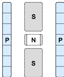
شکل ۲-۲۱- چیدمان H شکل
