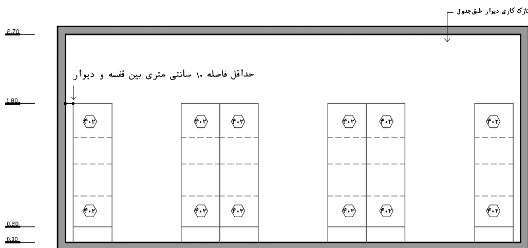
نقشه ۲-۱۳۶-۳- نمای ۳- مقیاس ۱:۵۰
