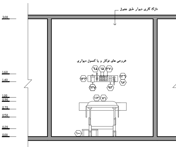
نقشه ۱-۴۳- نمای ۱- مقیاس ۱:۵۰
