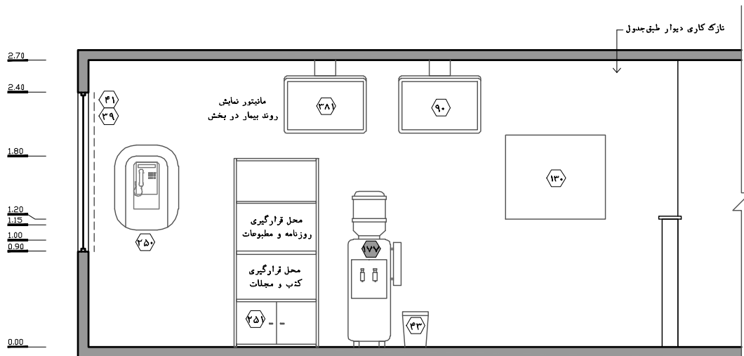
نقشه‌ی ۲-۹- نمای ۲- مقیاس ۱:۵۰
