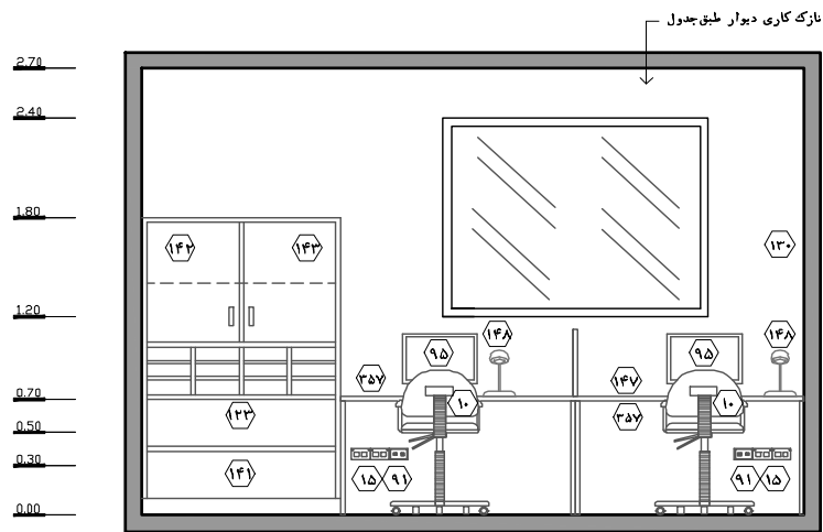
نقشه ۲-۱۲۷ - نمای ۱ - مقیاس ۱:۵۰
