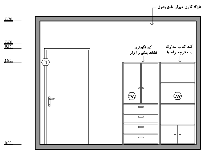
نقشه ۱۰۹-۲- نمای ۲- مقیاس ۱:۵۰
